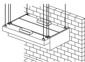
Plénum d'apport à rideau d'air (ASP)
