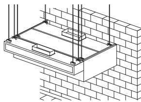
Plénum d'apport horizontal (HSP) Plénum d'apport variable (VSP)
